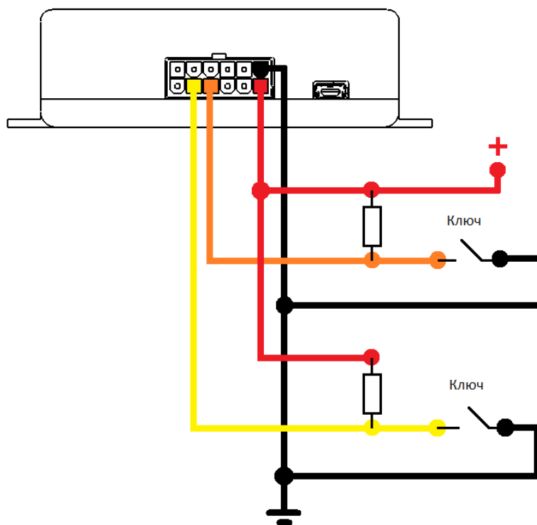
Рисунок 2.9 Подключение с подтяжкой к «+»
