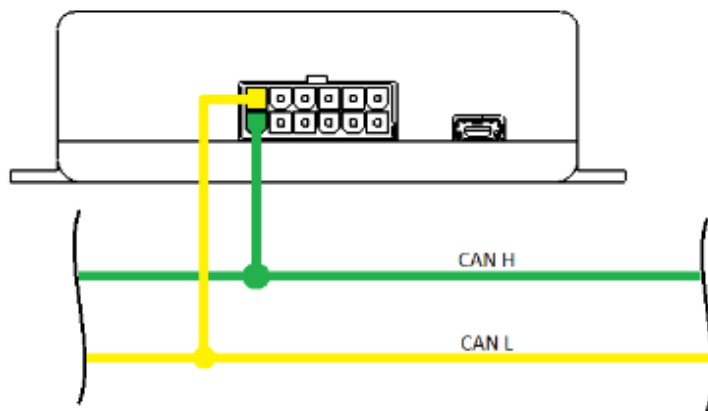
Рисунок 2.18 Подключение к шине CAN
