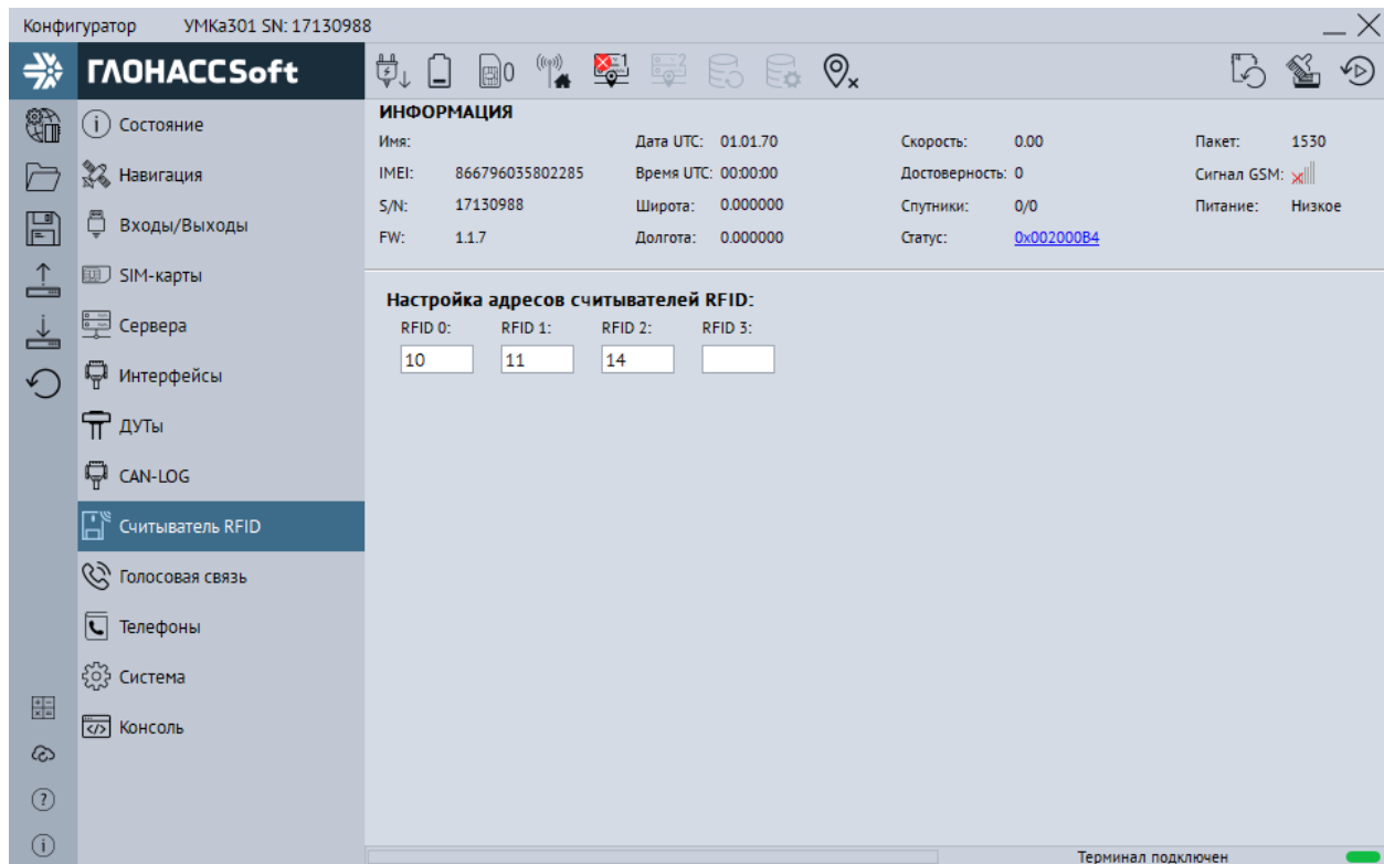
Рисунок 3.19 Вкладка «Считыватель RFID»
