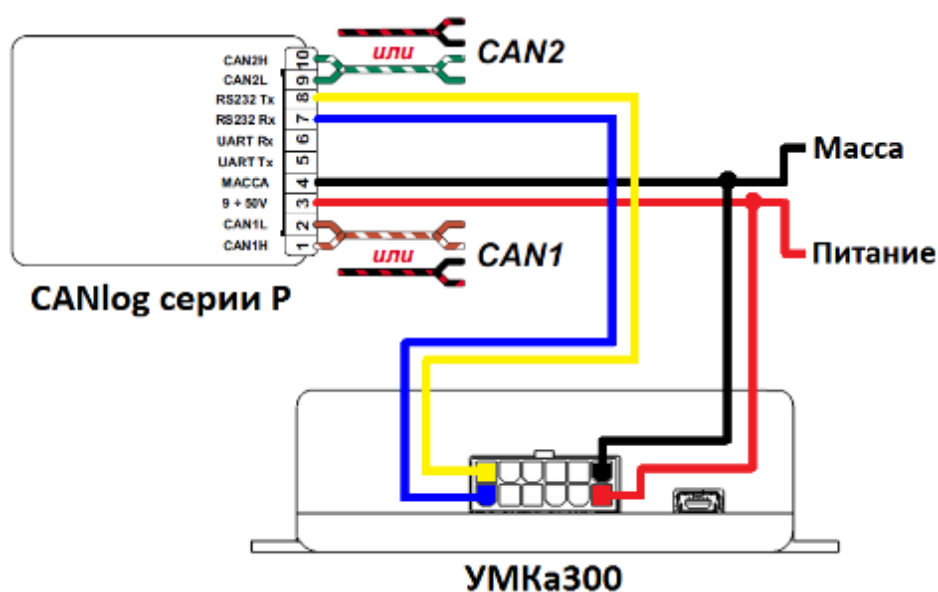
Рисунок 2.21 Подключение CAN-LOG по RS-232
