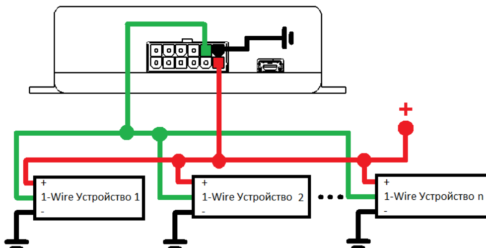
Рисунок 2.20 Подключение устройств по 1-Wire
