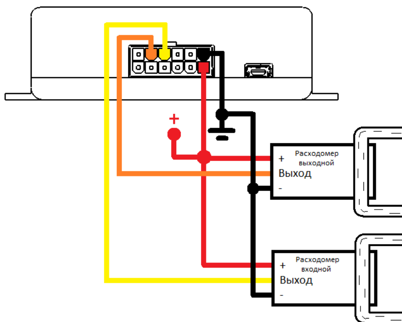
Рисунок 2.13 Пример подключения расходомеров в дифференциальном режиме
