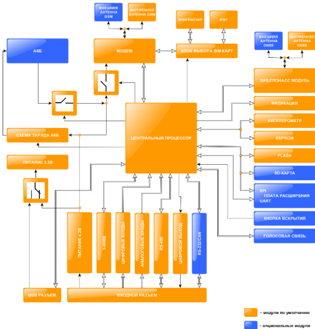
Рисунок 1.2 Блок-схема навигационного терминала
