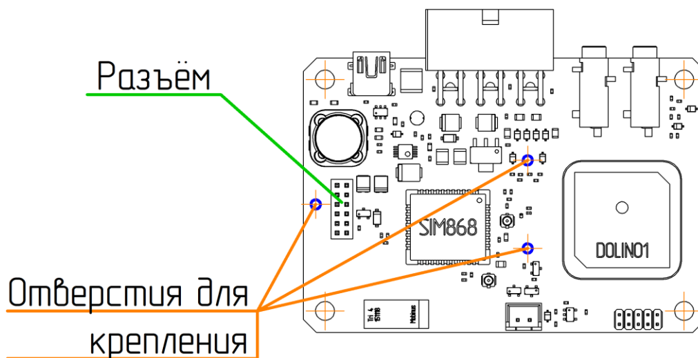
Рисунок 2.23 Место установки плат расширения
