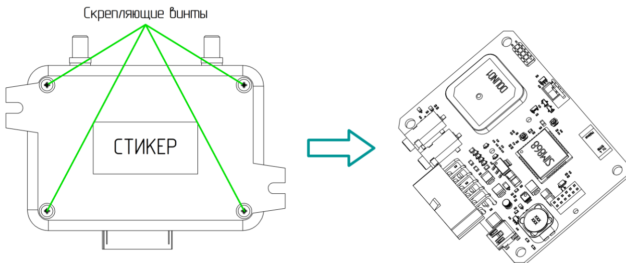
Рисунок 2.3 Вскрытие корпуса терминала
